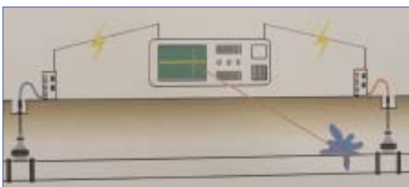
Schema Korrelationsverfahren.
